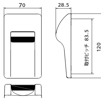
センサー部
